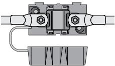
Fusible et porte-fusible simples fournis dans le Kit fusible REDARC référence FK40 (40A) ou FK60 (60A).
